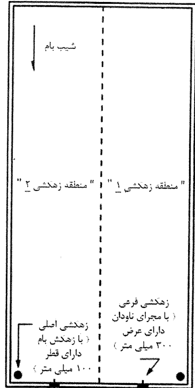
شکل ۶-۸-۱ دو نمونه شبکه زهکشی مجزا برای بام
