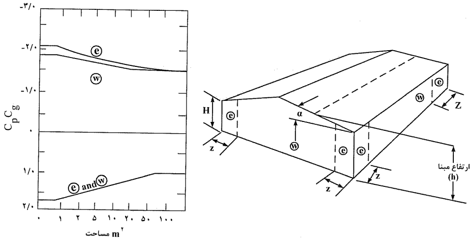
شکل ۳-۱۰-۶ ضرایب ترکیبی بیشینه فشار و باد جهشی خارجی، C_p C_g ، روی دیوارهای منفرد برای طراحی اجزاء سازه‌ای و پوسته خارجی و نما
