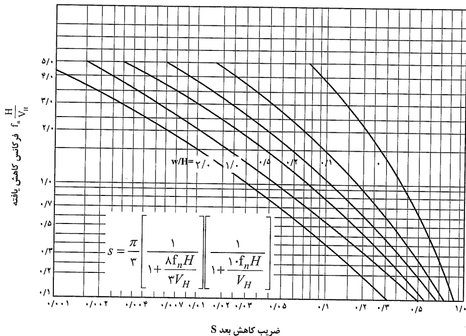
شکل پ-۶-۳ ضریب کاهش ابعادی بعنوان تابع عرض به ارتفاع و کاهش فرکانس سازه
